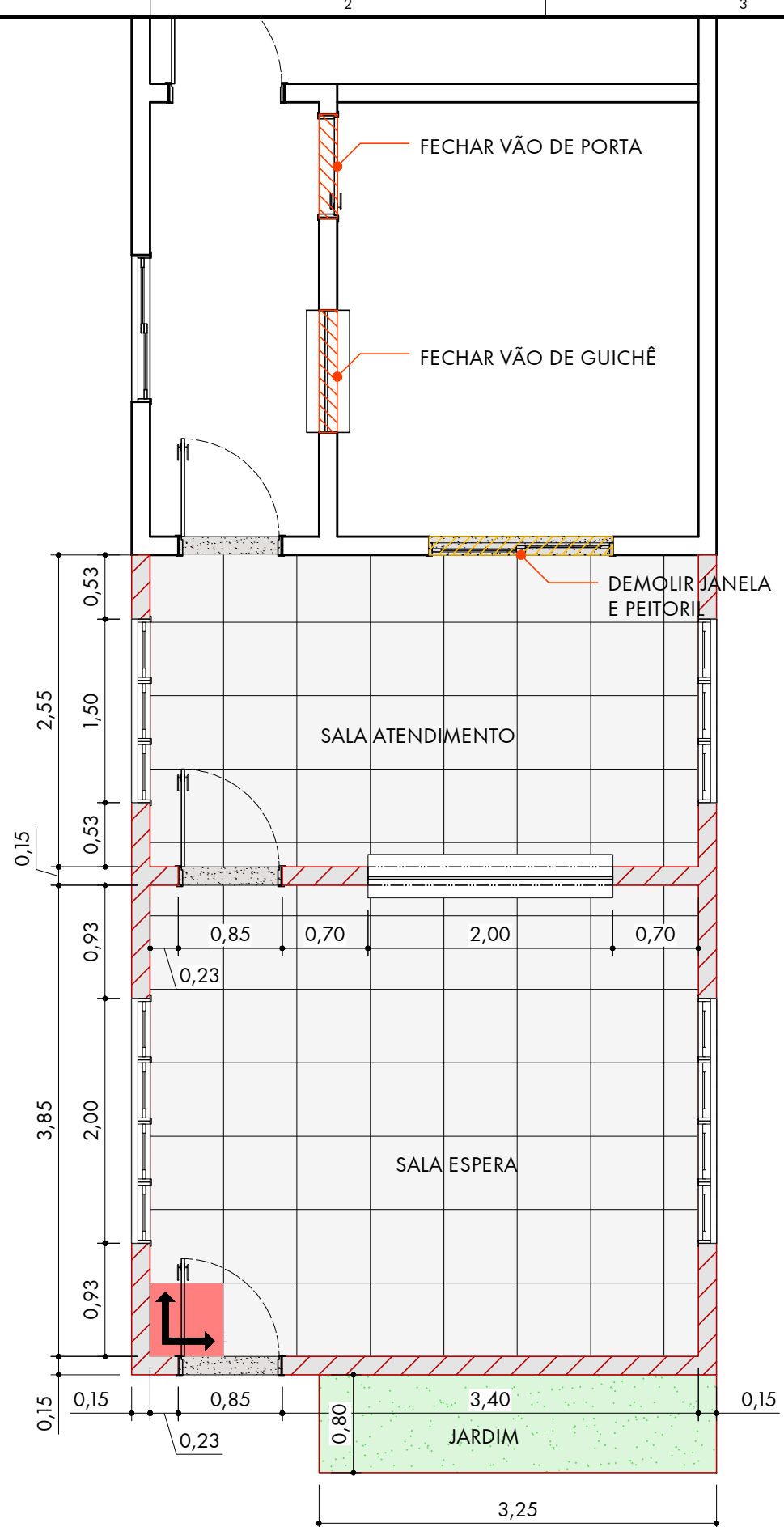
1 PLANTA BAIXA 1:50
